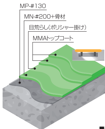
■ペースト工法(2mm)
