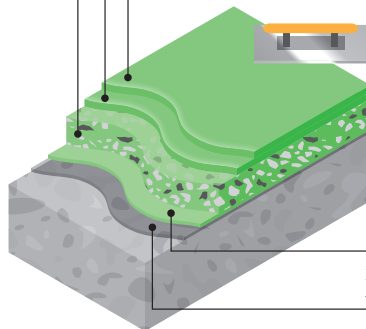
■樹脂モル工法(5mm)
