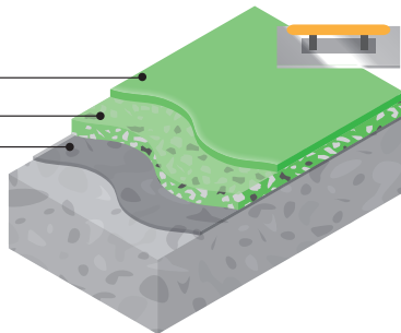
■ペースト工法(2mm)
