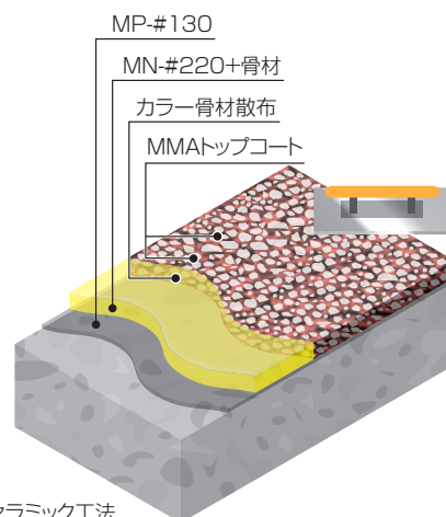
■カラーセラミック工法 防滑仕上材(3mm)
